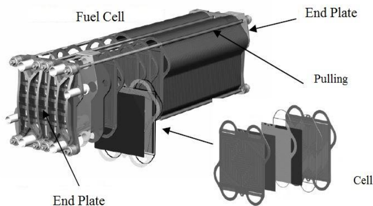
Figure 8 : Exemple d'un assemblage de pile à combustible [19]
